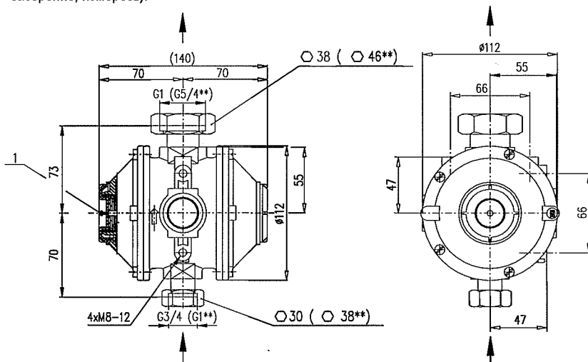
RTP ..-М.-Р с прямыми вводами и с перекидной гайкой
